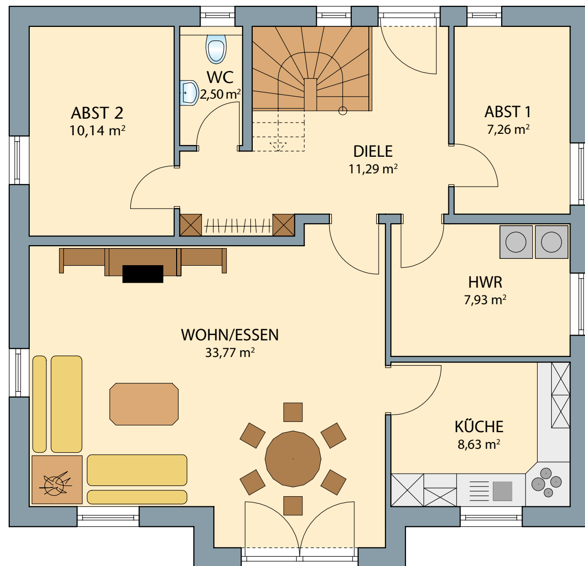
➤ Grundriss Erdgeschoss
