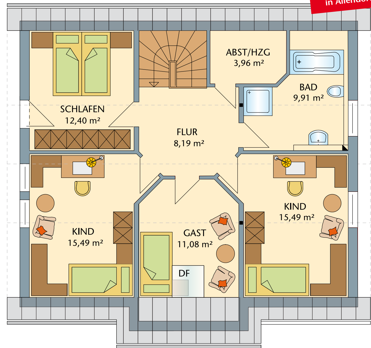
➤ Grundriss Dachgeschoss
